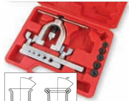
Single Flare Double Flare
