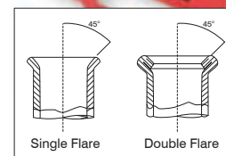
Single Flare Double Flare
